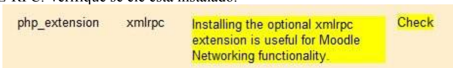
Xmlrpc_check.jpg
