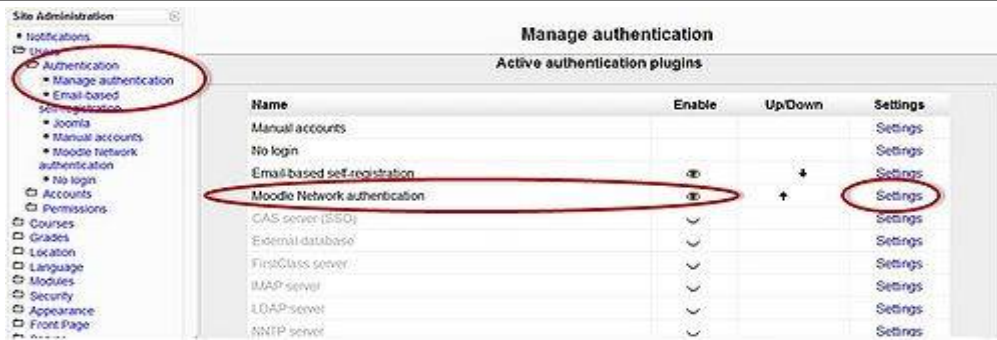
500px-R023_moodle_config_network_authentication_1.jpg
